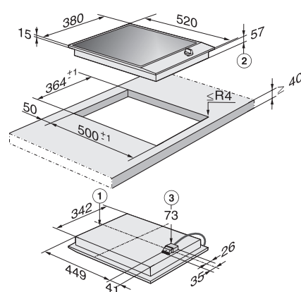
Plan de cuisson à induction CS 1222 I
