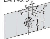
Hotte aspirante murale DAH 4970
