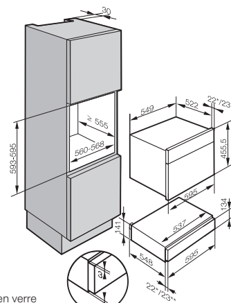
Tiroir Sous vide EVS 7010 en combinaison avec four compact
